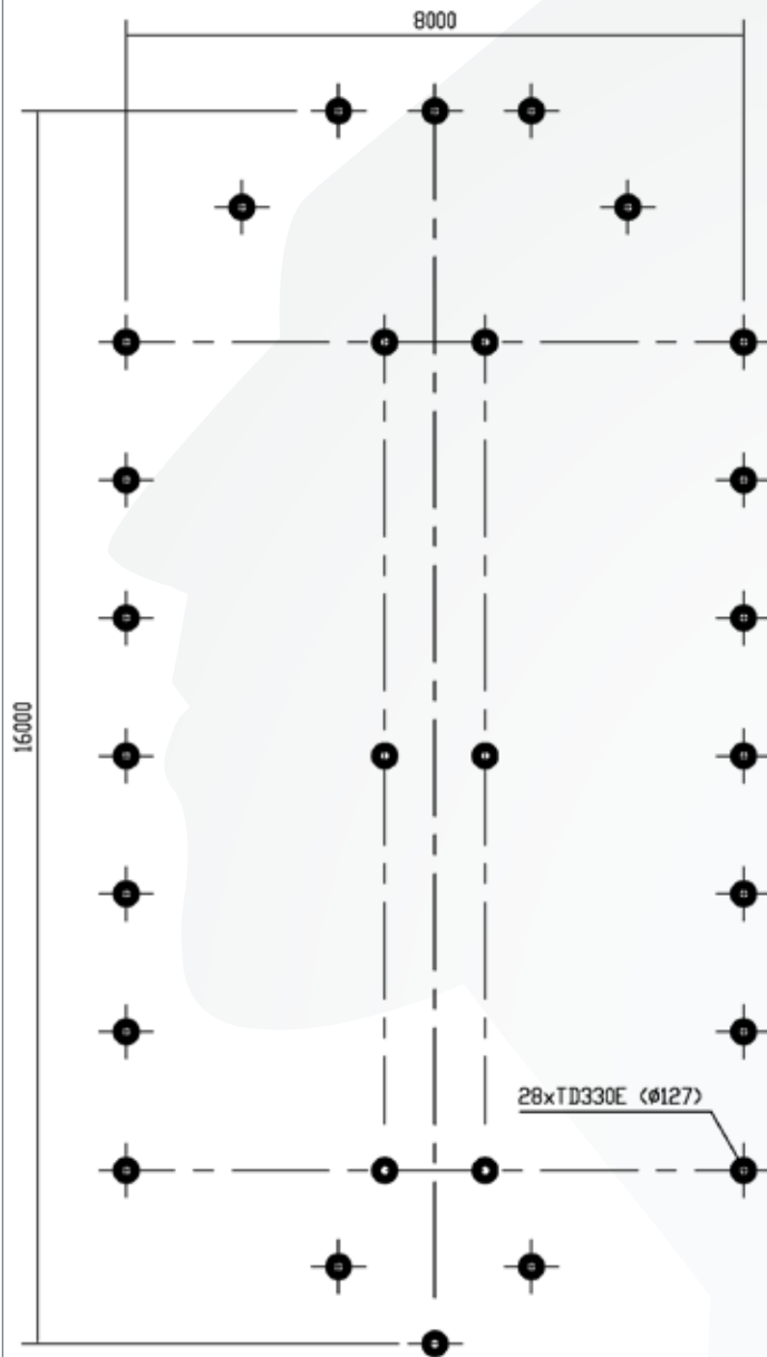
16 M X 8 M TD 330E / TD130E
