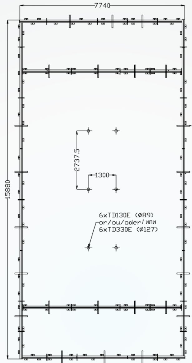
KOREK® KOR85B + KOR71B - 16 M X 8 M TD 330E / TD130E
